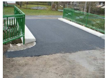
Rekonstrukce mostů přes Novoveský potok
